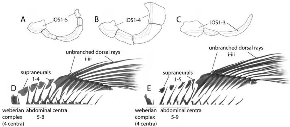
FIGURE 3. Isolated infraorbital series: A , E. walshae (AMNH 266860); B , E. camptacanthus (AMNH 256416); C , E. jae (AMNH 253857). Anterior vertebrae, dorsal fin, and associated supra-neuronal elements; D , E. walshae (AMNH 266862); E , E. catenarius (AMNH 266868).
