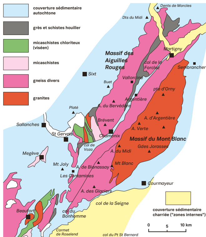
Fig. 1. – Carte géologique synoptique de la zone d'étude avec les massifs cristallins et les hautes chaînes calcaires des nappes helvétiques. [Carte modifiée d'après GIDON (2020)]
