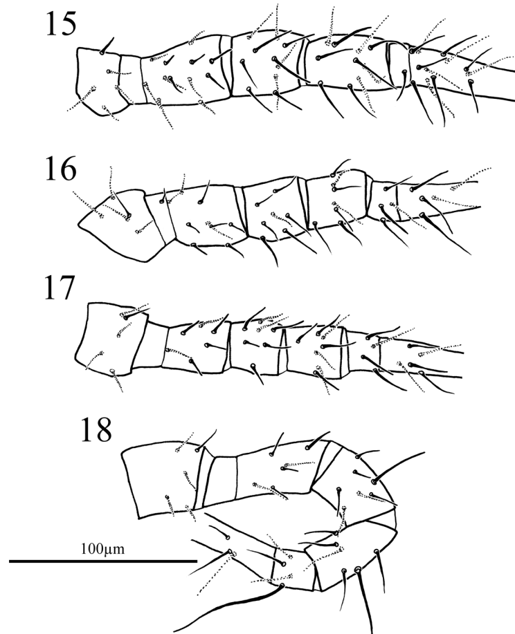
FIGURES 15–18. Neoseiulus xiaomenensis sp. nov. , female, legs (trochanter–basitarsus). 15. Leg I; 16. Leg II; 17. Leg III; 18. lLeg IV.
