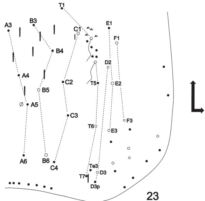
Fig. 23. Lepidonella marimuti , dorsal chaetotaxy of abdomen 4.
