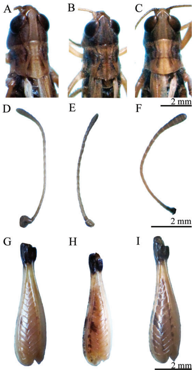
Fig. 3. Pronotum head, antennae, and hind femur of males of R. turcicus populations. (A, D, G) Türbe. (B, E, H) Uluğaç. (C, F, I) Yarılgöz.
