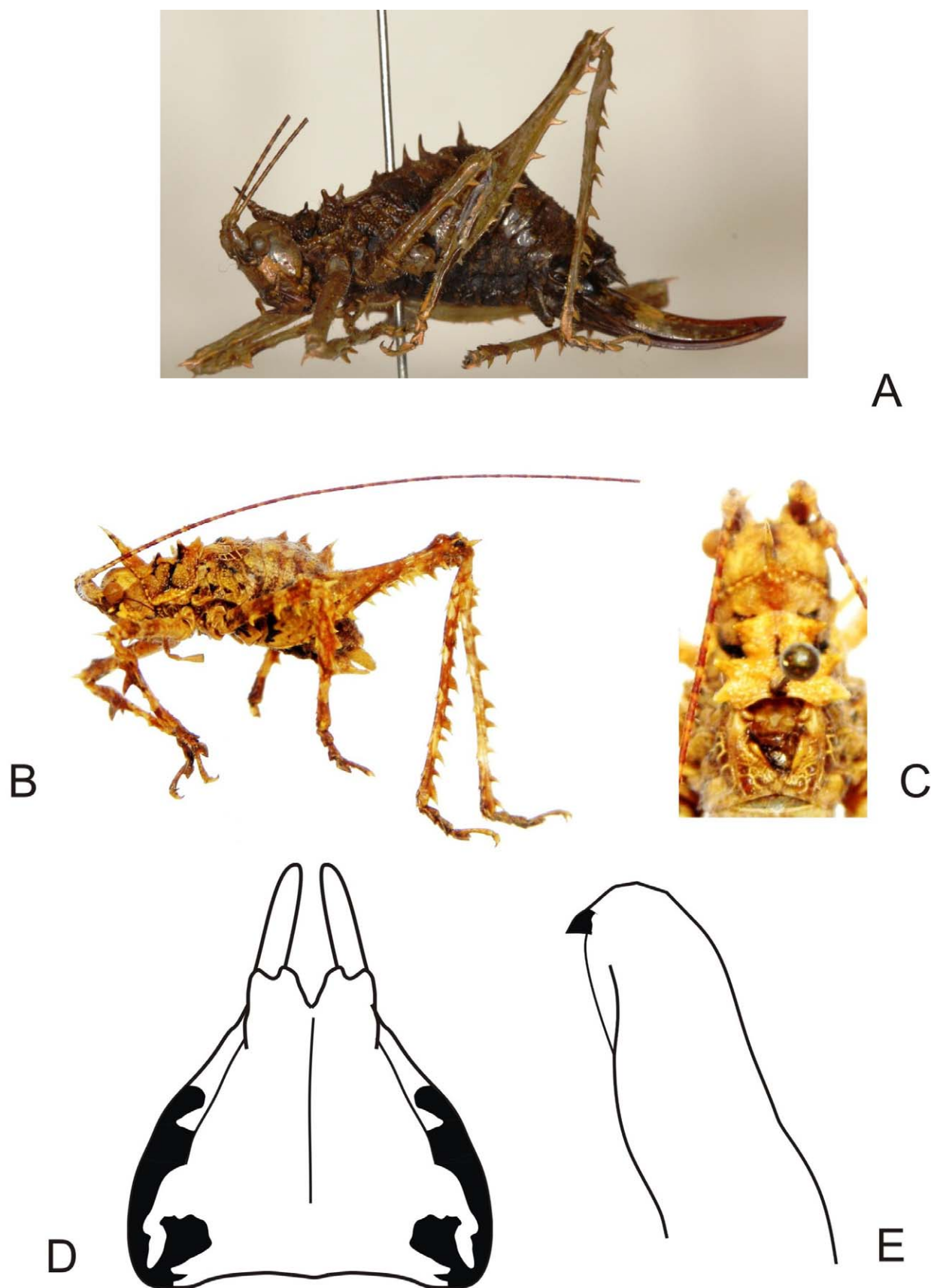
Fig. 1. (A-E) Adeclus spiculatus . A. Habitus de la hembra, B. Habitus del macho, C. Pronoto y tegmina del macho en vista dorsal, D. Placa subgenital, E. Cerco en vista dorsal.
