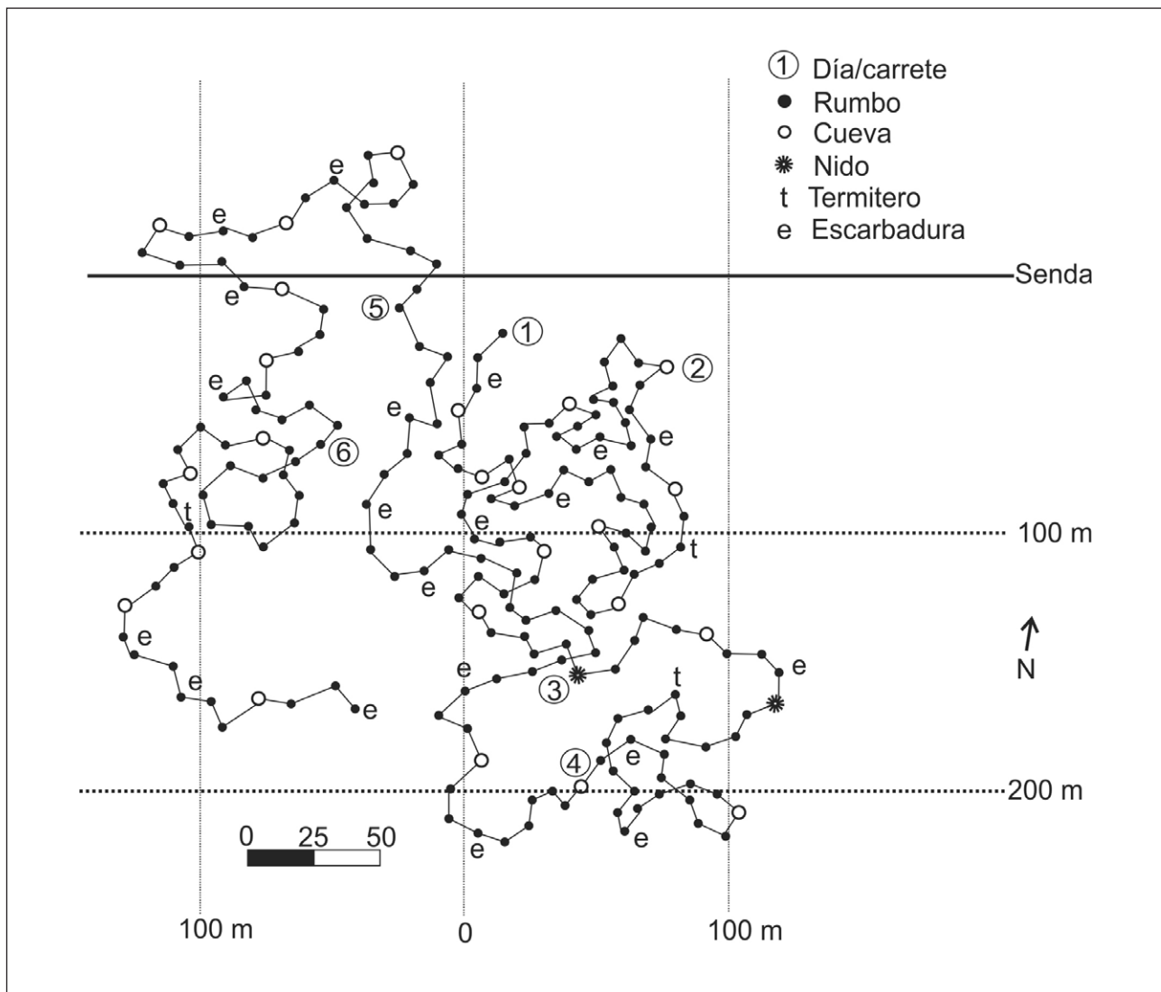
FIGURA 2. Mapa del seguimiento por hilos de Tolypeutes matacus en Cerro Cortado, Chaco boliviano. Macho N° 26: 4 días, 1.370 m de recorrido, S_1=15,31 , S_2=1,37 ; 21 escarbadoras; 3 termiteros; 24 cuevas; 2 nidos (Modificado de Enrique Perrogón, cuaderno de campo). Para más datos ver TABLA 1 . S_1 =Recorrido total/Distancia entre punto inicial y punto final, S_2 =Largo/Ancho del área de acción durante los 1-5 días de seguimiento. Rumbo=Sitio donde se determinó el rumbo del siguiente trayecto de 10 m aproximados.
